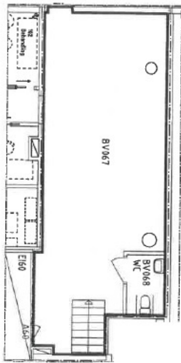
Plan 3, bottenvåning
