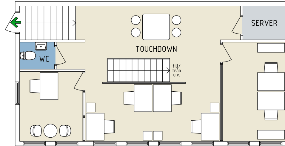
ÖVERVÅNING LOKALAREA CA 71 KVM
