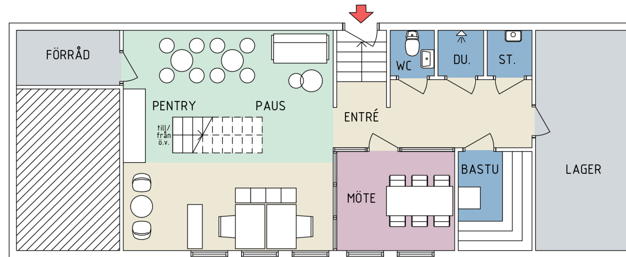
UNDERVÅNING LOKALAREA CA 87 KVM
